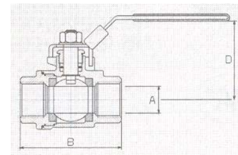
Рис. 2. Шаровой кран, тип 2BV2HFT
